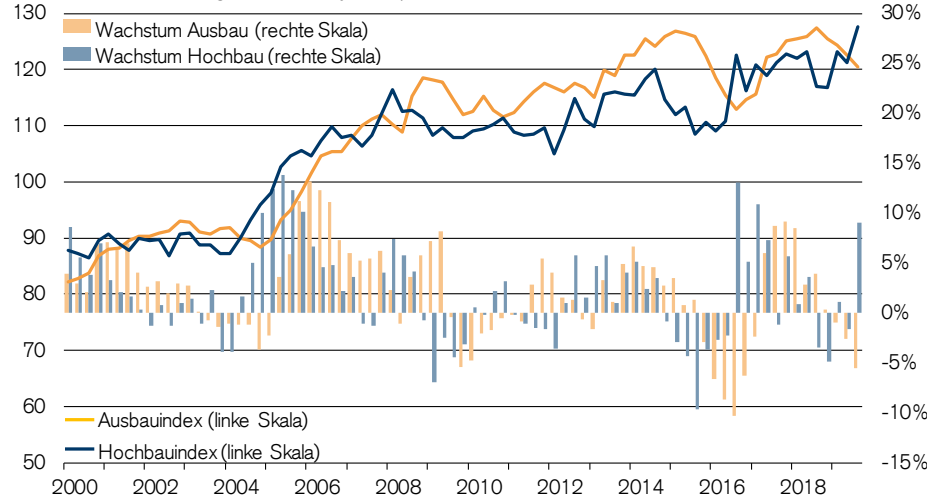
Ausbau- und Hochbauindex 1.Q. 1996 = 100, saisonbereinigt, nominal; Wachstumsraten im Vergleich zum Vorjahresquartal
