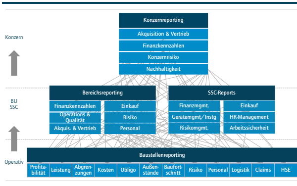
Abb. 11: Exemplarische Reportingstruktur
